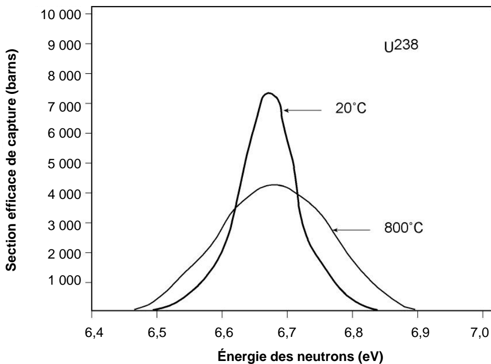
Figure 21.2 Élargissement des résonances
